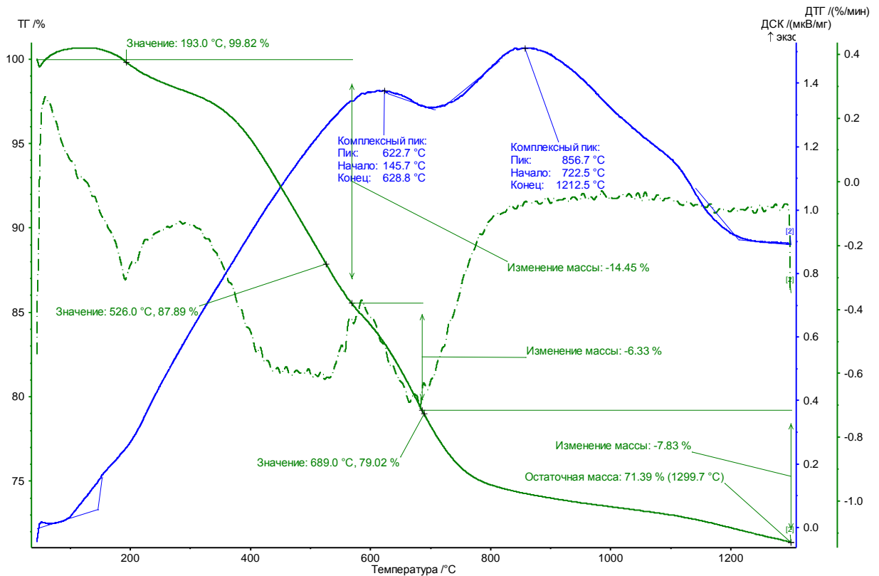
Рисунок 3.68 – Кривые ТГ и ДСК Та/ZrKC с. 2
