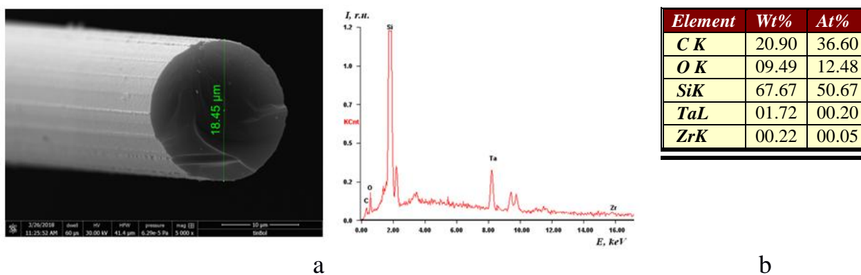
Рисунок 3.79 – Микрофотография и рентгеновский элементный микроанализ волокна Ta/ZrKC–1250(Ar)
