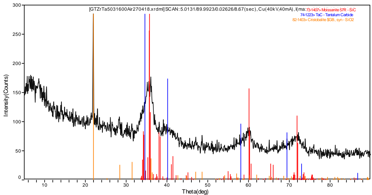
Рисунок 12 – Дифрактограмма образца керамики с. 1–1600(Air)
