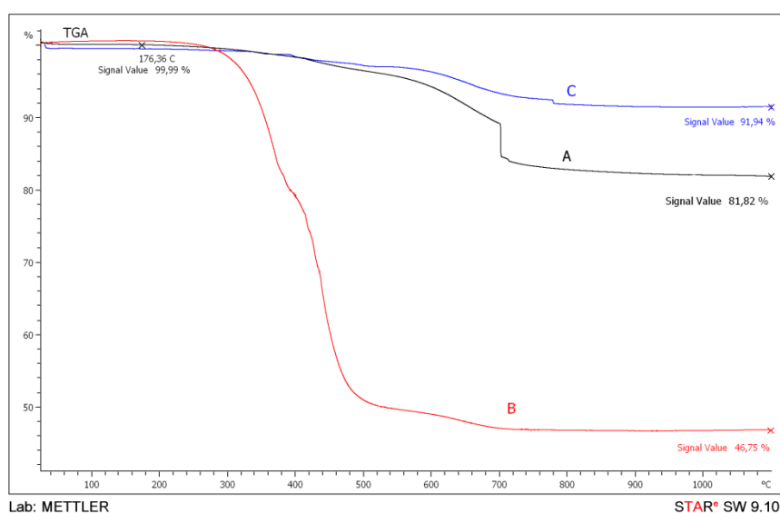
Рисунок 3.26 – Кривые ТГА образцов НfКС с содержанием гафния более 5 мас. % в атмосфере аргона до 1100 °С: А – с. 3; В – с. 4; С – с. 14
