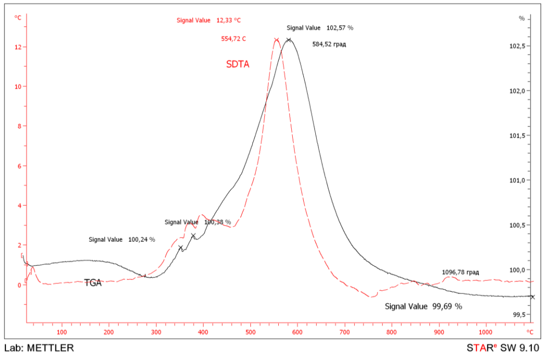
Рисунок 3.30 – Кривые ТГА и SDTA HfKС с. 3 до 1100 °С на воздухе
