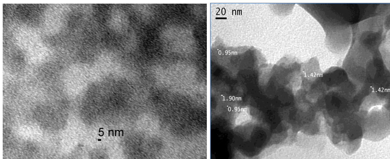
Рисунок 3.54 – Микрофотография ПЭМ с. 1 ТаКС (табл. 3.15)
