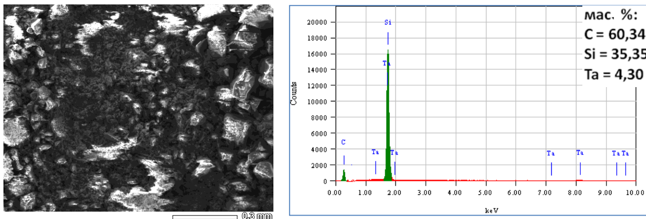
Рисунок 3.53 – Микрофотографии СЭМ и рентгеновский элементный микроанализ с. 3 ТаКС (табл. 3.15)
