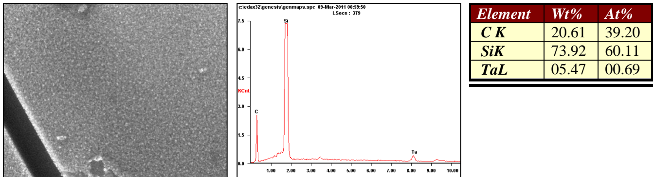
Рисунок 3.60 – Результаты СЭМ и рентгеновский элементный микроанализ керамики с. 1 ТаКС–1100(Ar)
