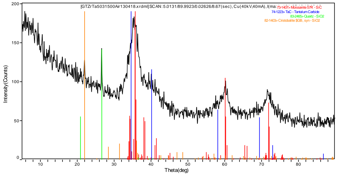
Рисунок 11 – Дифрактограмма образца керамики с. 1–1500(Air)
