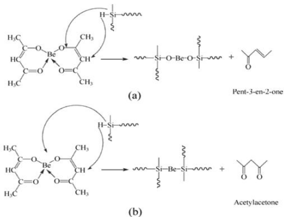
Рисунок 1.6 – Механизм реакции ПКС с \text{Be}(\text{acac})_2 [57]
