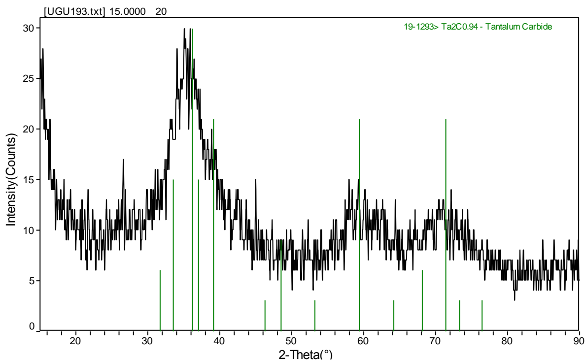
Рисунок 3.61 – Типичная дифрактограмма образца керамики ТаКС–1100(Аг)
