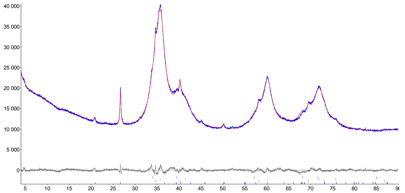
Рисунок 1 – Дифрактограмма образца керамики с. 1–1500(N 2 )
