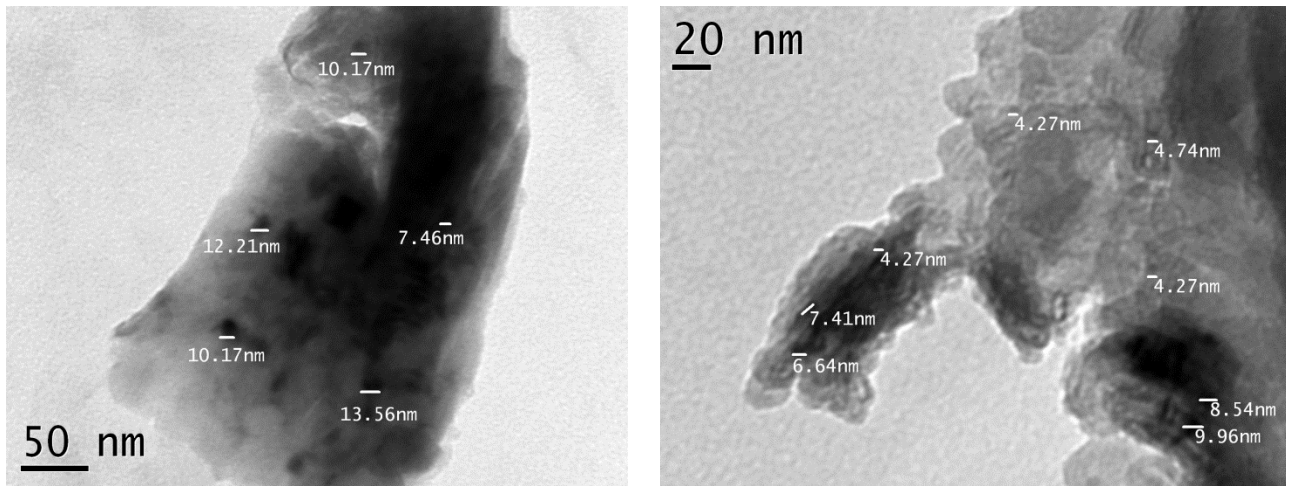
Рисунок 3.59 – Микрофотографии образца керамики с. 1 ТаКС–1100(Ar)
