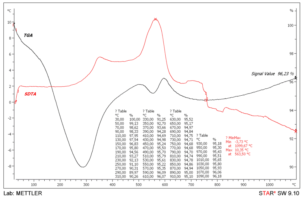
Рисунок 3.32 – Кривые ТГА и SDTA HfKС с. 14 до 1100 °C на воздухе
