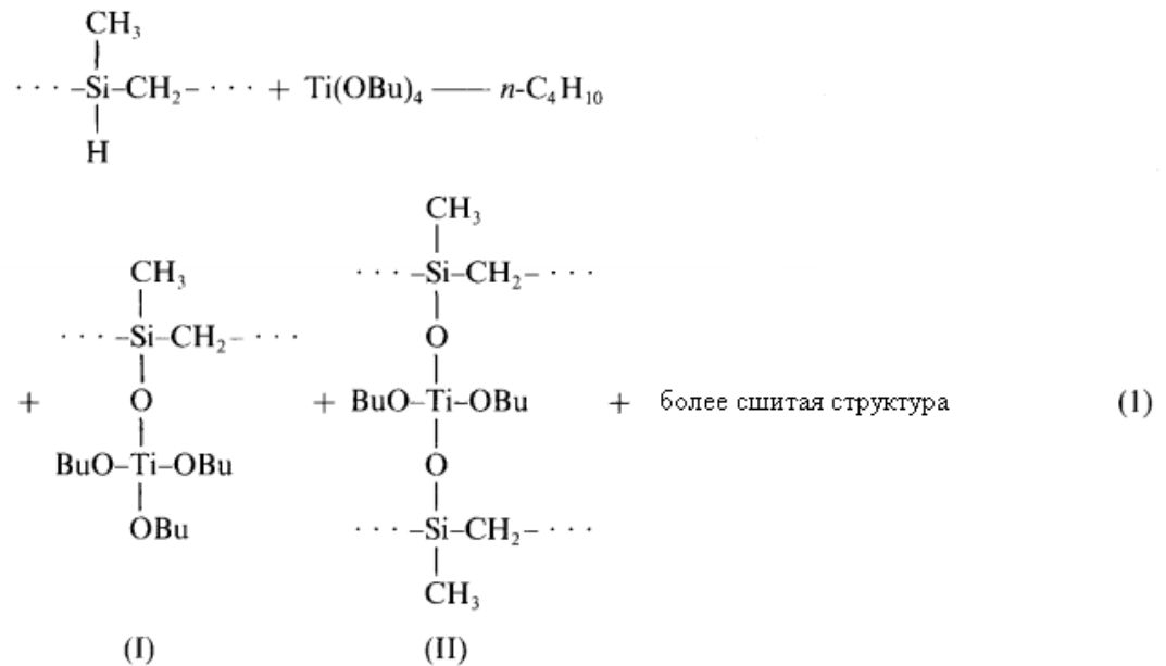
Рисунок 1.2 – Синтез TiПКС из тетрабутоксид титана и ПКС [35]
