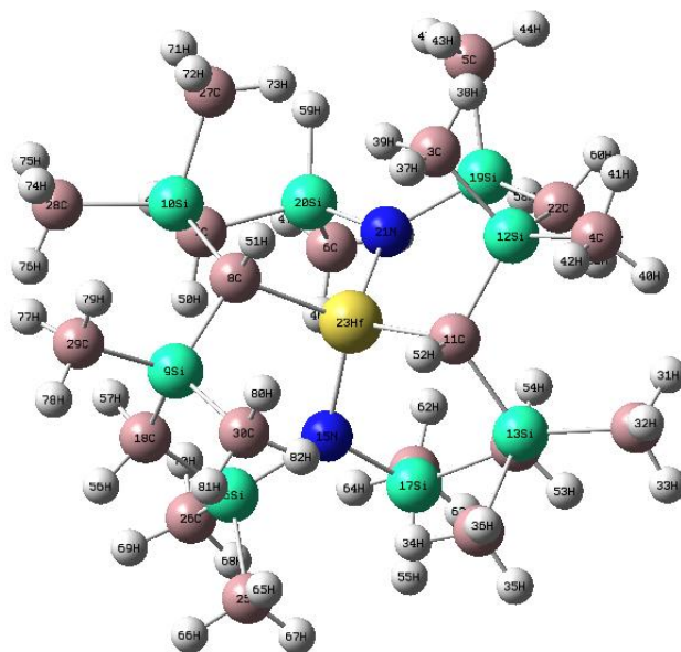
Рисунок 3.24 – Вероятная молекулярная структура гафнийсодержащего олигомера 1 типа (HfKC с. 6) C_{19}H_{52}N_2Si_8Hf : а – проекция 1; б – проекция 2; с – проекция 3
