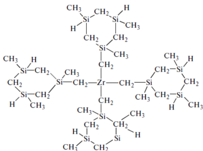
Рисунок 3.14 – Вероятное строение нано-ZrОКС-2 (1 тип) [98]
