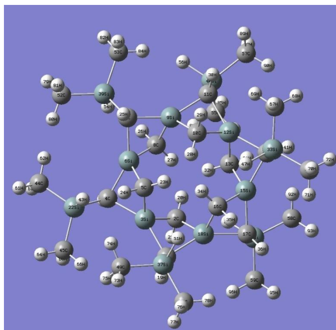
Рисунок 3.9 – Молекулярная структура поликарбосилана C_{25}H_{64}Si_{12} (проекция 1) [186]
