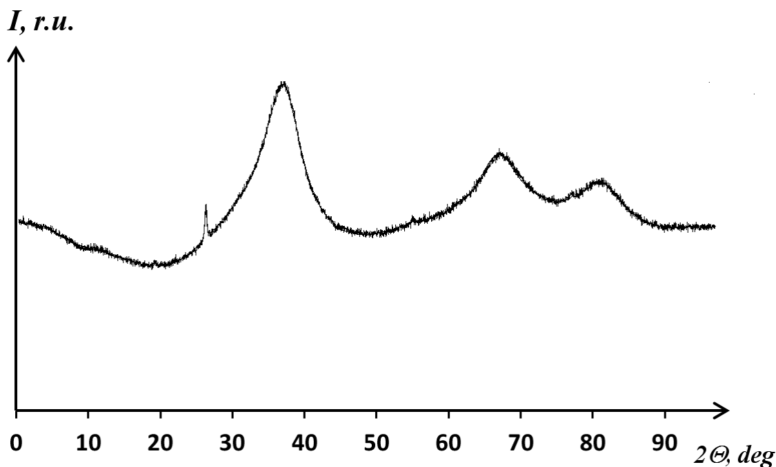
Рисунок 3.80 – Дифрактограмма волокна Ta/ZrKC–1250(Ar)
